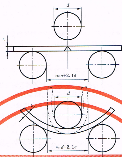
图 6 对接接头弯曲试验
